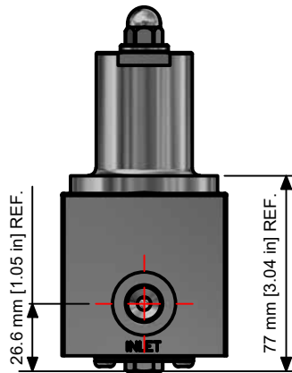
Seitl. Ansicht
